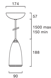
CDM-TC & QT12-LPax
